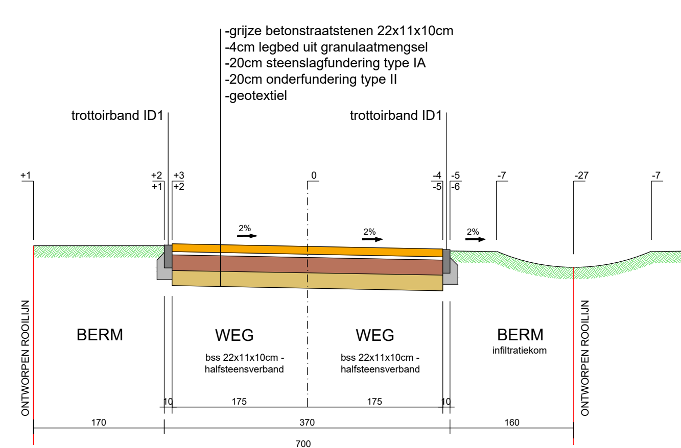
TYPEDWARSPROFIEL L-L
