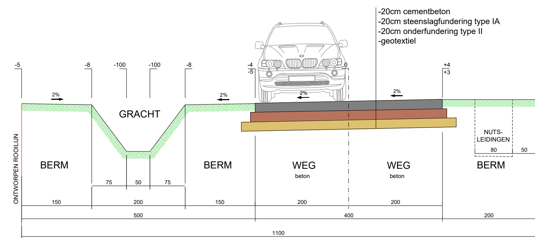
TYPEDWARSPROFIEL I-I
