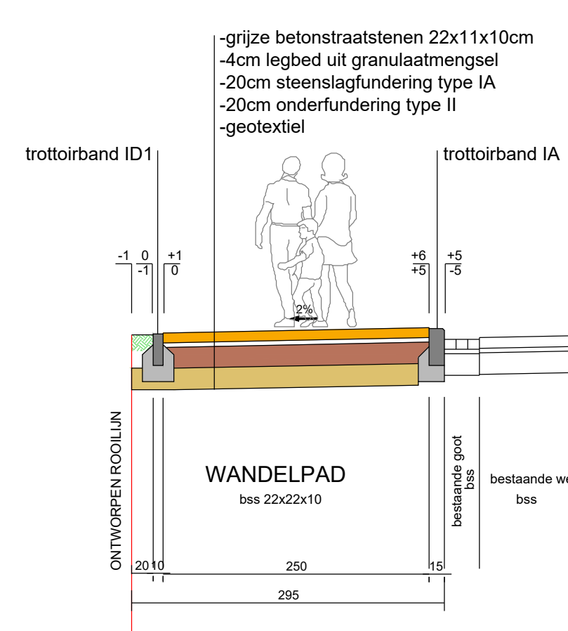
TYPEDWARS E-E
