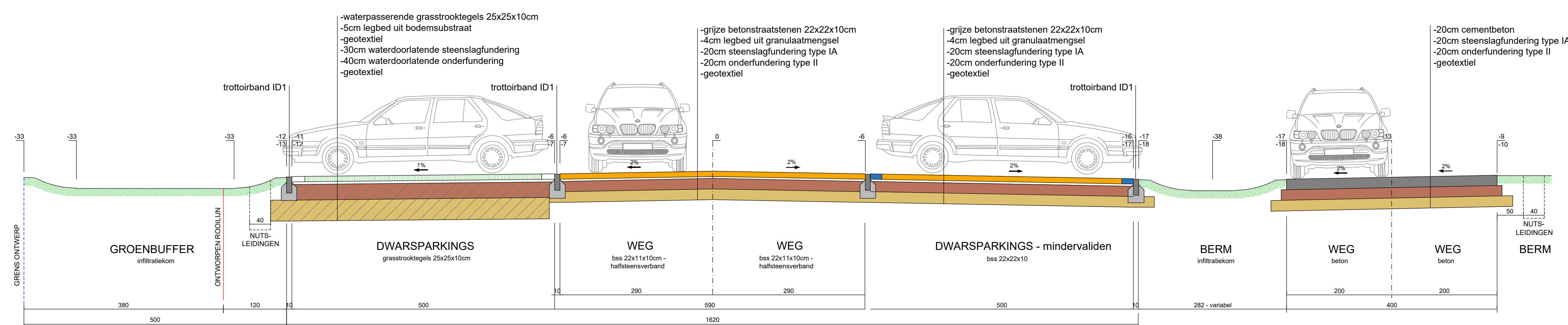
TYPEDWARSPROFIEL G-G
