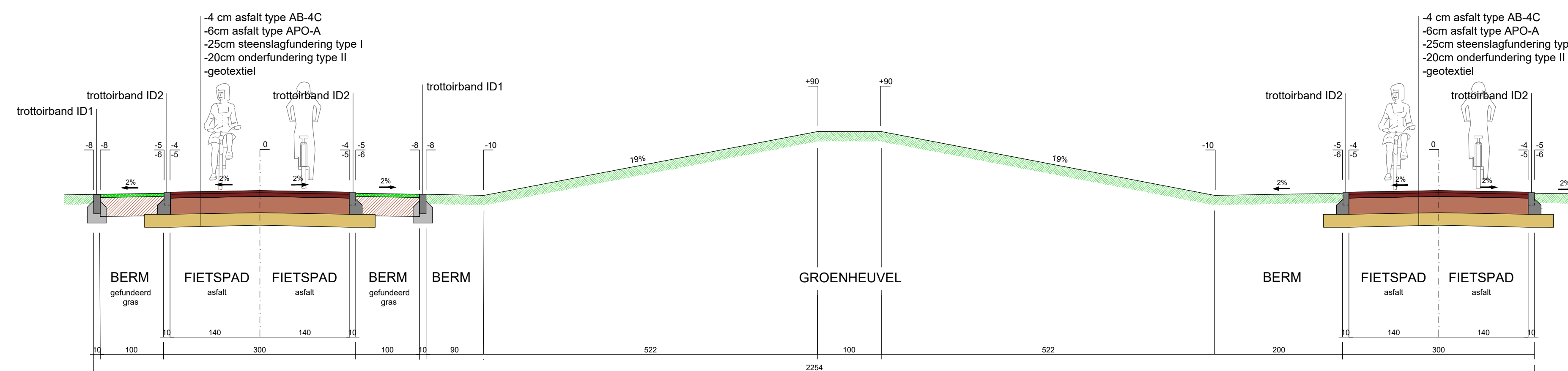
TYPEDWARSPROFIEL K-K
