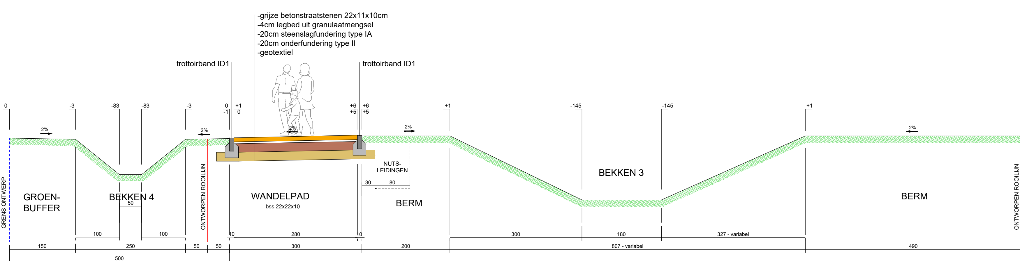
TYPEDWARSPROFIEL F-F
