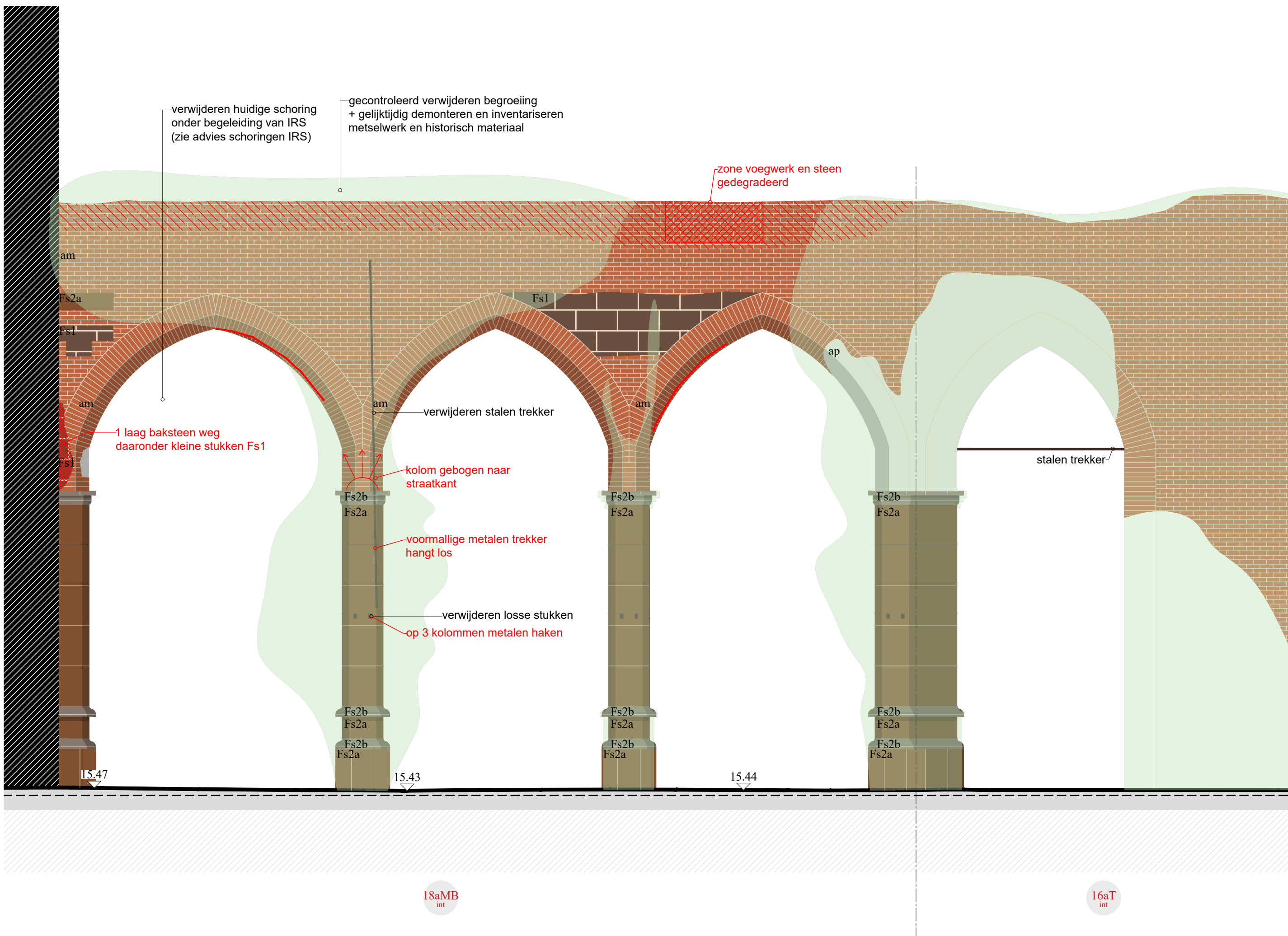
ONTWIKKELING MIDDENBEUK
