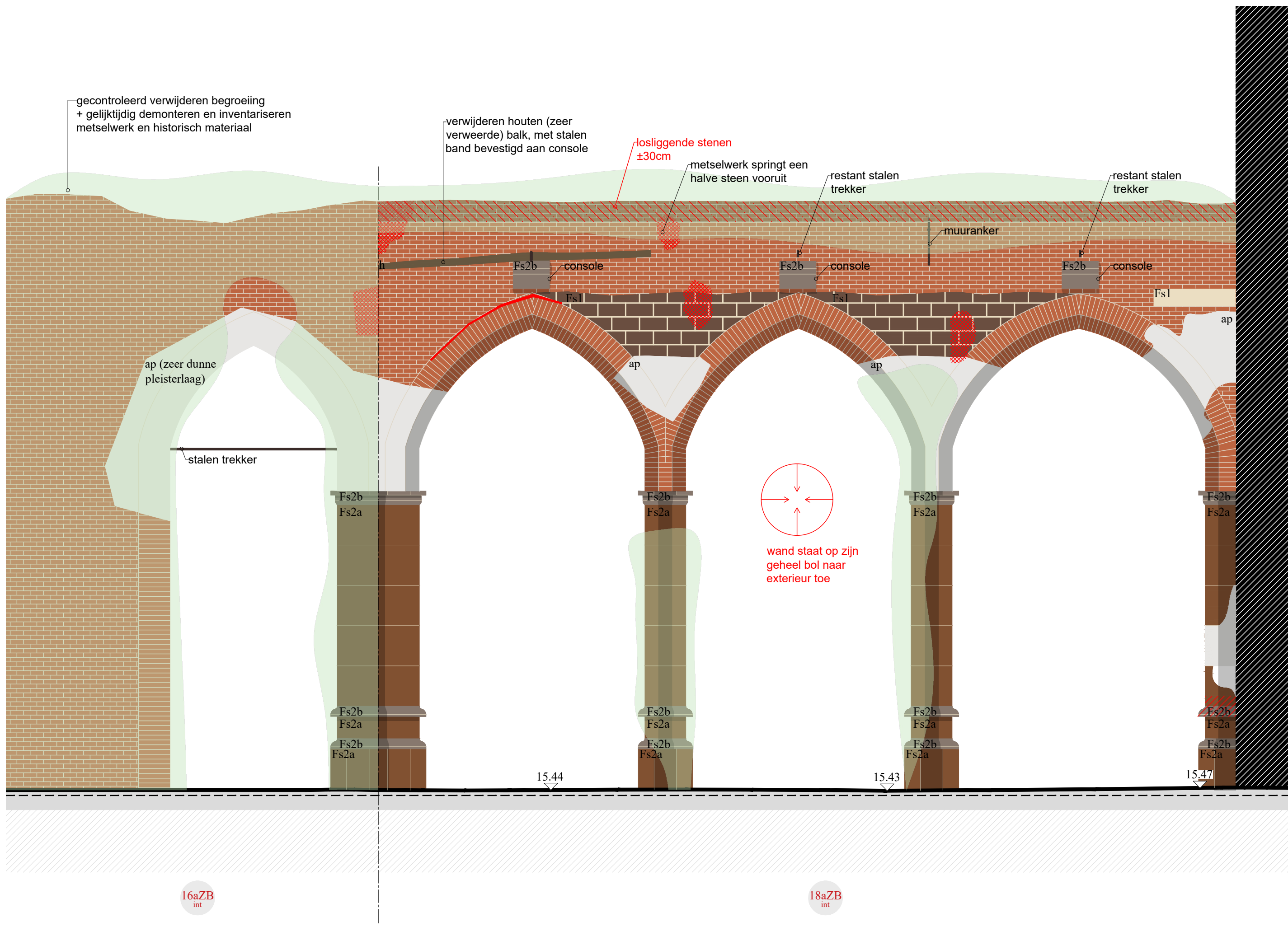
ONTWIKKELING ZIJBEUK
