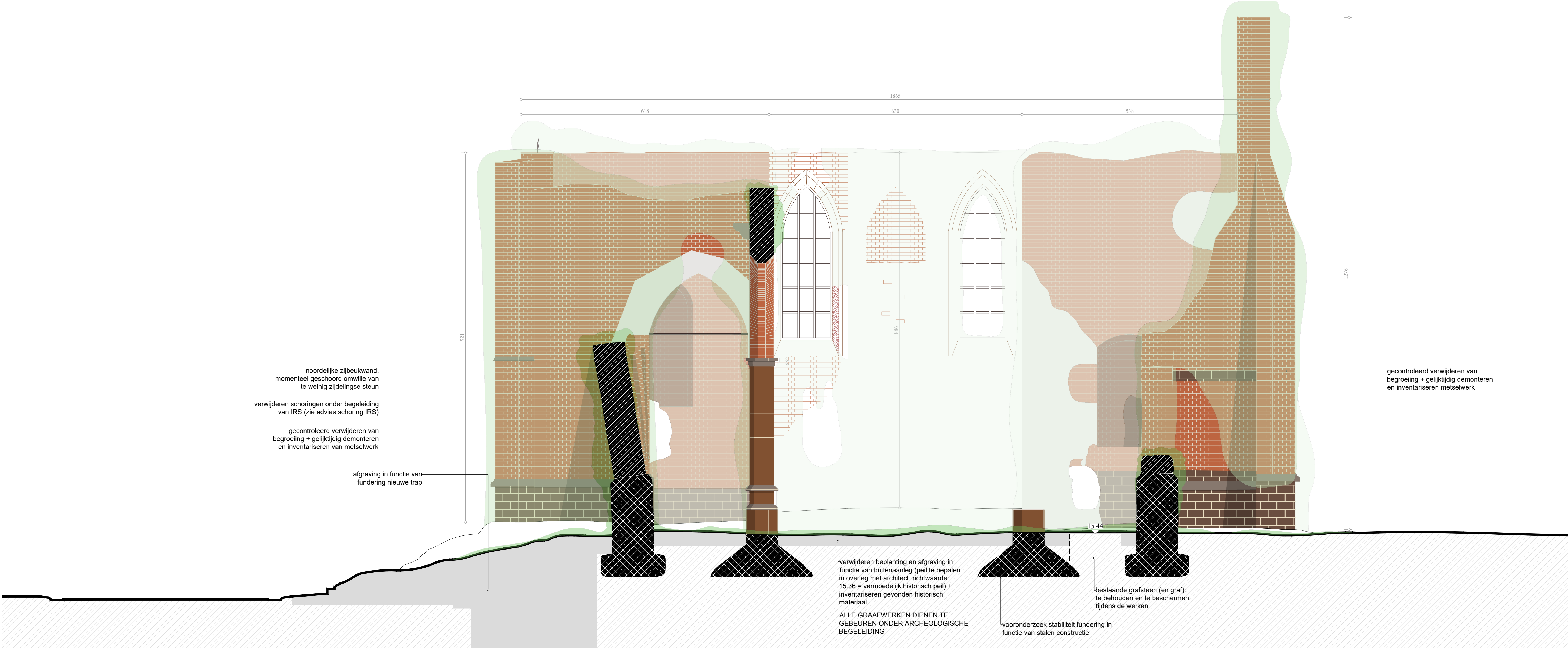
DOORSNEDE A
