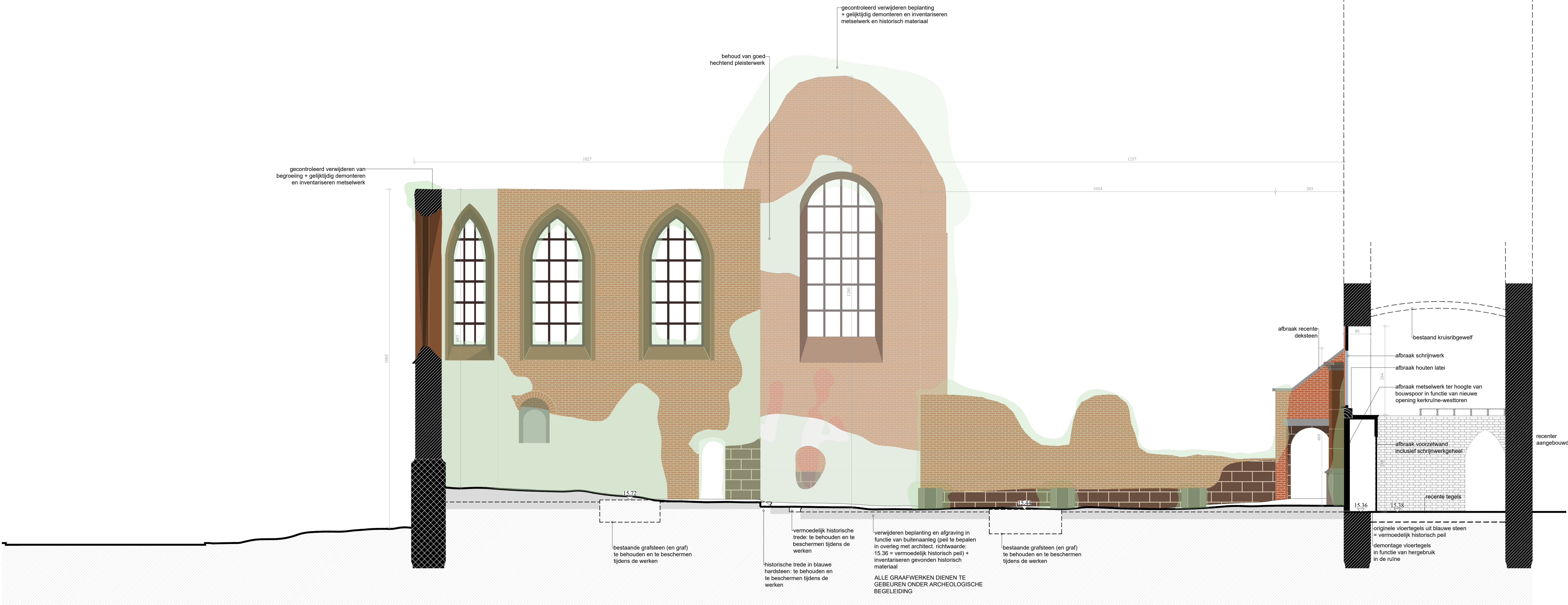
DOORSNEDE B
